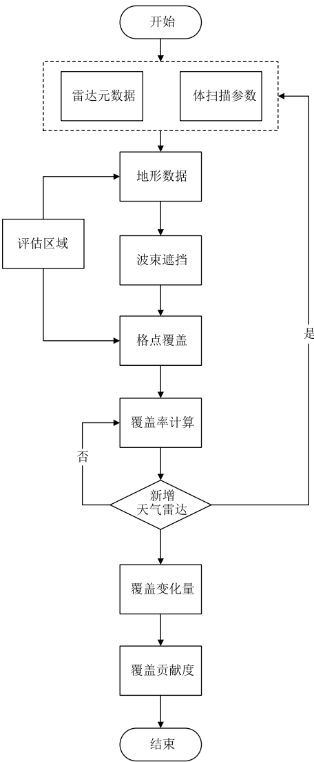
图 1 天气雷达覆盖率和贡献度计算方法流程
