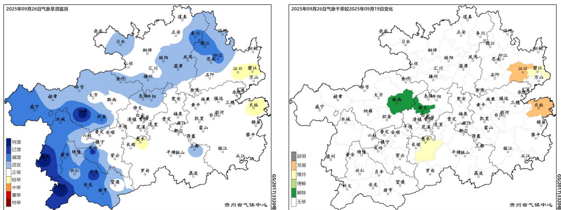
图 3 贵州省 2025 年 9 月 26 日气象旱涝综合监测及其与 9 月 19 日对比
