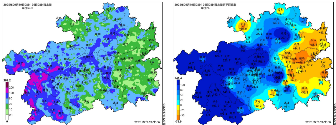
图2 贵州省2025年9月19日08时—26日08时降水量及其距平百分率分布
