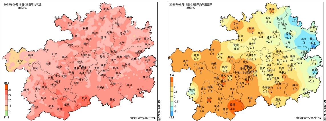
图1 贵州省2025年9月19日—25日平均气温及其距平分布
