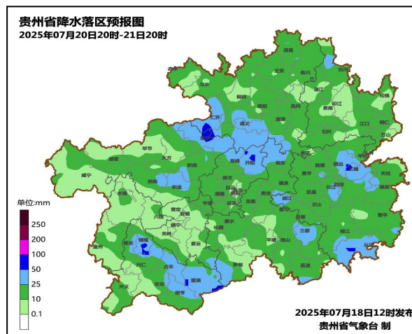
图3 贵州省2025年7月20日20时至21日20时降水落区预报图
