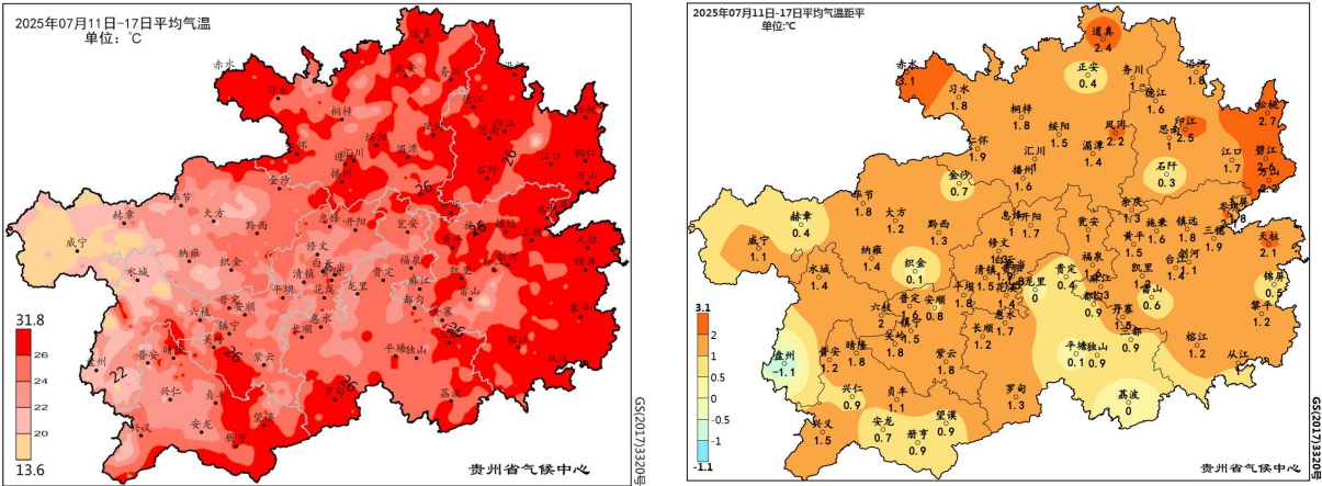
图 4 贵州省 2025 年 7 月 11 日至 17 日平均气温及其距平分布
