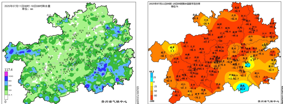
图5 贵州省2025年7月11日08时至18日08时降水量及其距平百分率分布
