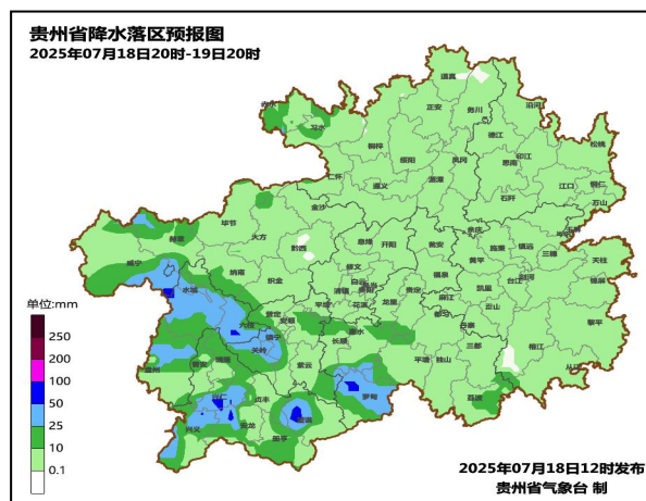
图1 贵州省 2025 年 7 月 18 日 20 时至 19 日 20 时降水落区预报图
