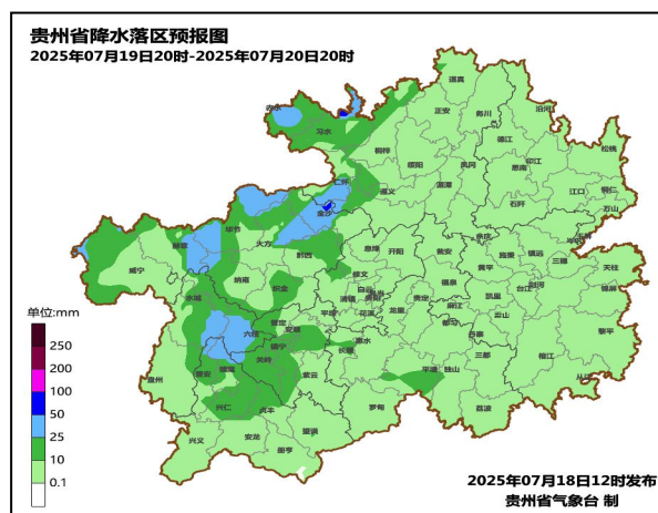
图2 贵州省 2025 年 7 月 19 日 20 时至 20 日 20 时降水落区预报图
