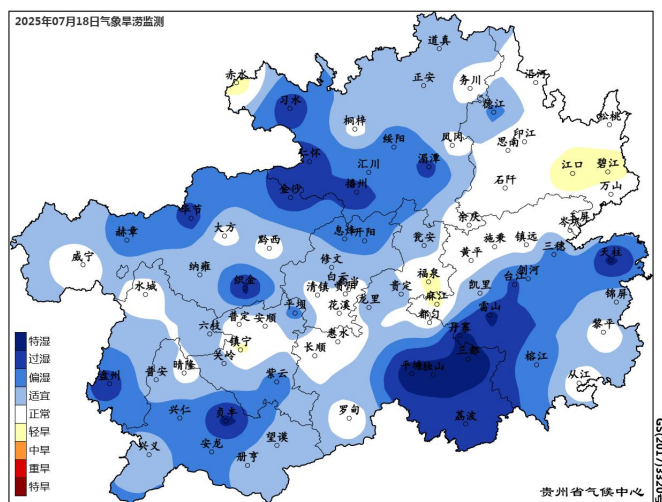
图6 贵州省2025年7月18日气象旱涝综合监测
