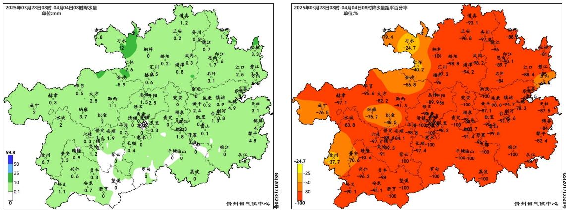
图2 贵州省2025年3月28日08时-4月4日08时降水量及其距平百分率分布
