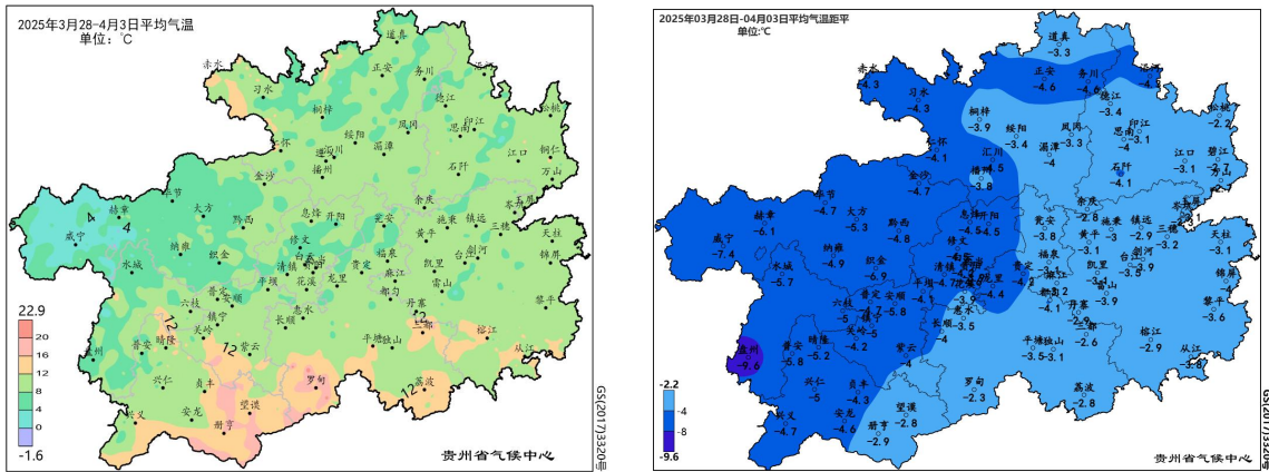
图1 贵州省2025年3月28日-4月3日平均气温及其距平分布
