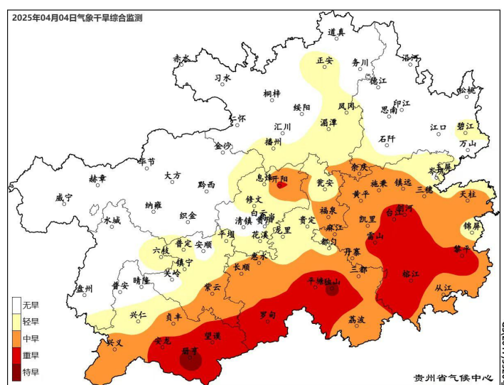
图3 贵州省2025年4月4日气象旱涝监测
