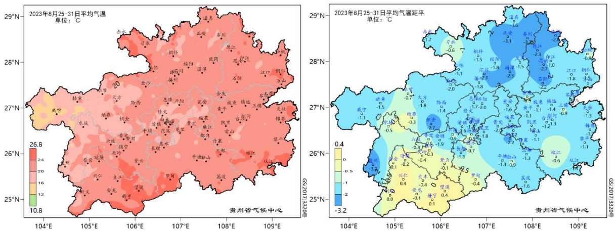
图1 贵州省2023年8月25日-8月31日平均气温及其距平分布
