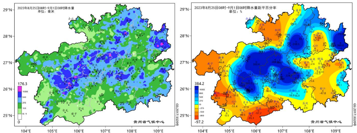
图2 贵州省2023年8月25日08时-9月1日08时降水量及其距平分布
