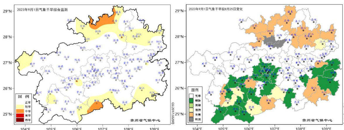
图3 贵州省2023年9月1日气象干旱综合监测及其与8月25日对比
