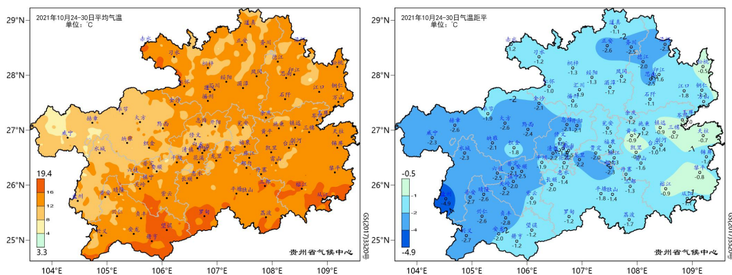
图 1 贵州省 2021 年 10 月 24-30 日平均气温及其距平分布
