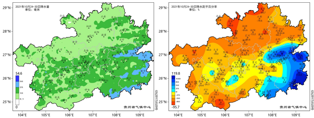
图 2 贵州省 2021 年 10 月 24-30 日降水量及其距平百分率分布
