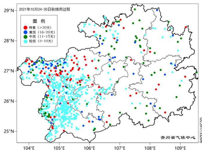
图4 贵州省2021年24-30日秋绵雨过程情况
