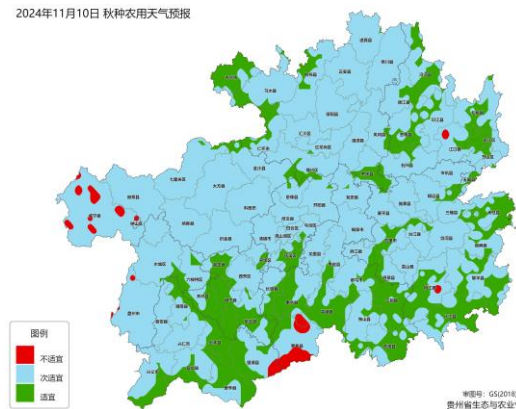
图2 未来4天贵州省秋种适宜气象等级分布图
