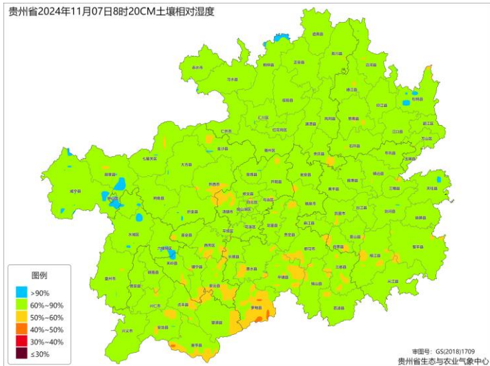
图 1 贵州省 2024 年 11 月 7 日土壤相对湿度图
