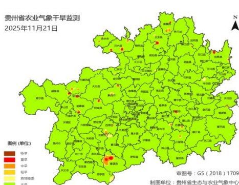
图 7 贵州省 11 月 21 日 (左) 与 11 月 28 日 (右) 农业气象干旱对比
