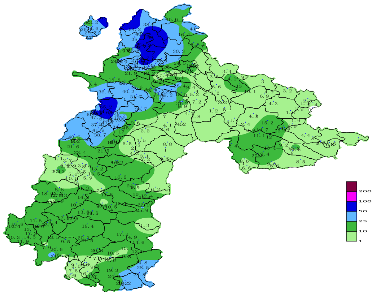
六盘水市2024092008-2024092708降雨量
