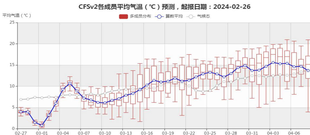
图 1 2024 年 2 月 26 日~4 月 9 日平均气温预测
