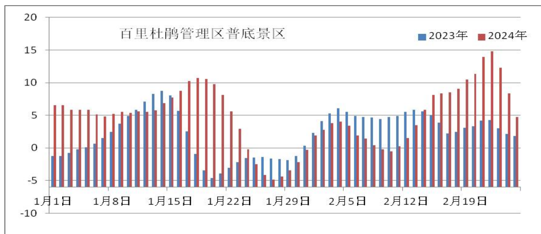
图3 2023、2024年1月1日~2月25日百里杜鹃景区气温变化图
