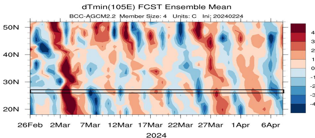
图2 2024年2月26日~4月9日冷空气影响过程预测
